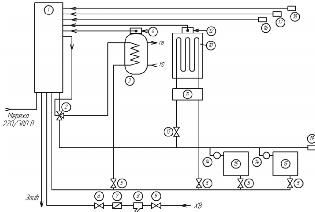
Рекомендована схема системи опалення
