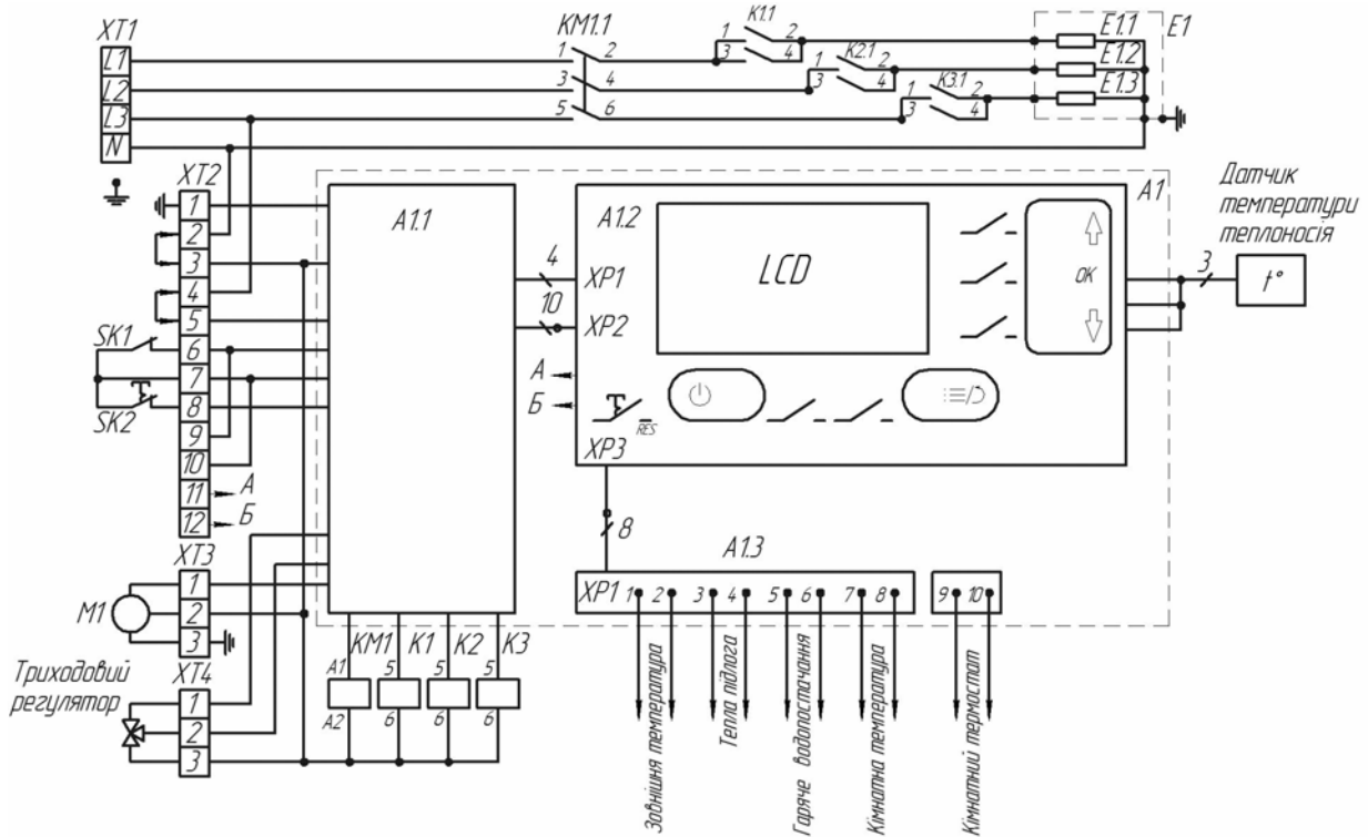
Рекомендована схема системи опалення
